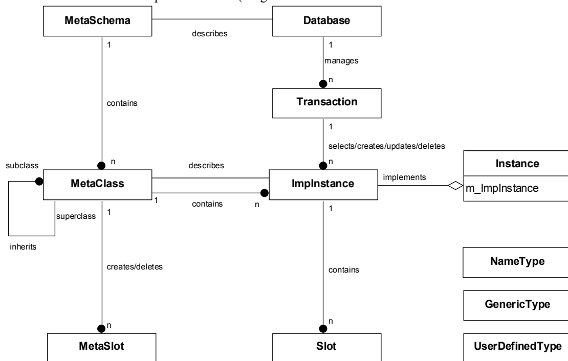
Bild 1: Klassendiagramm der AKO-Schnittstelle
