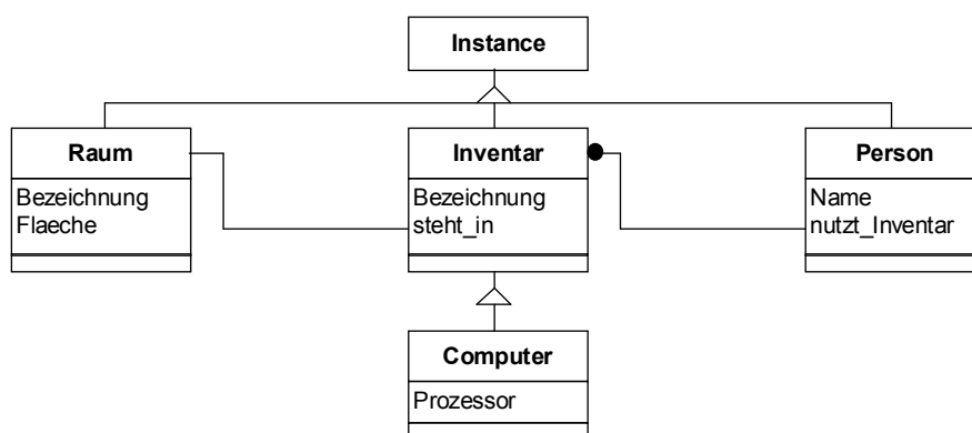
Bild 2: Einfache Klassenhierarchie für eine Facility-Management-Anwendung
