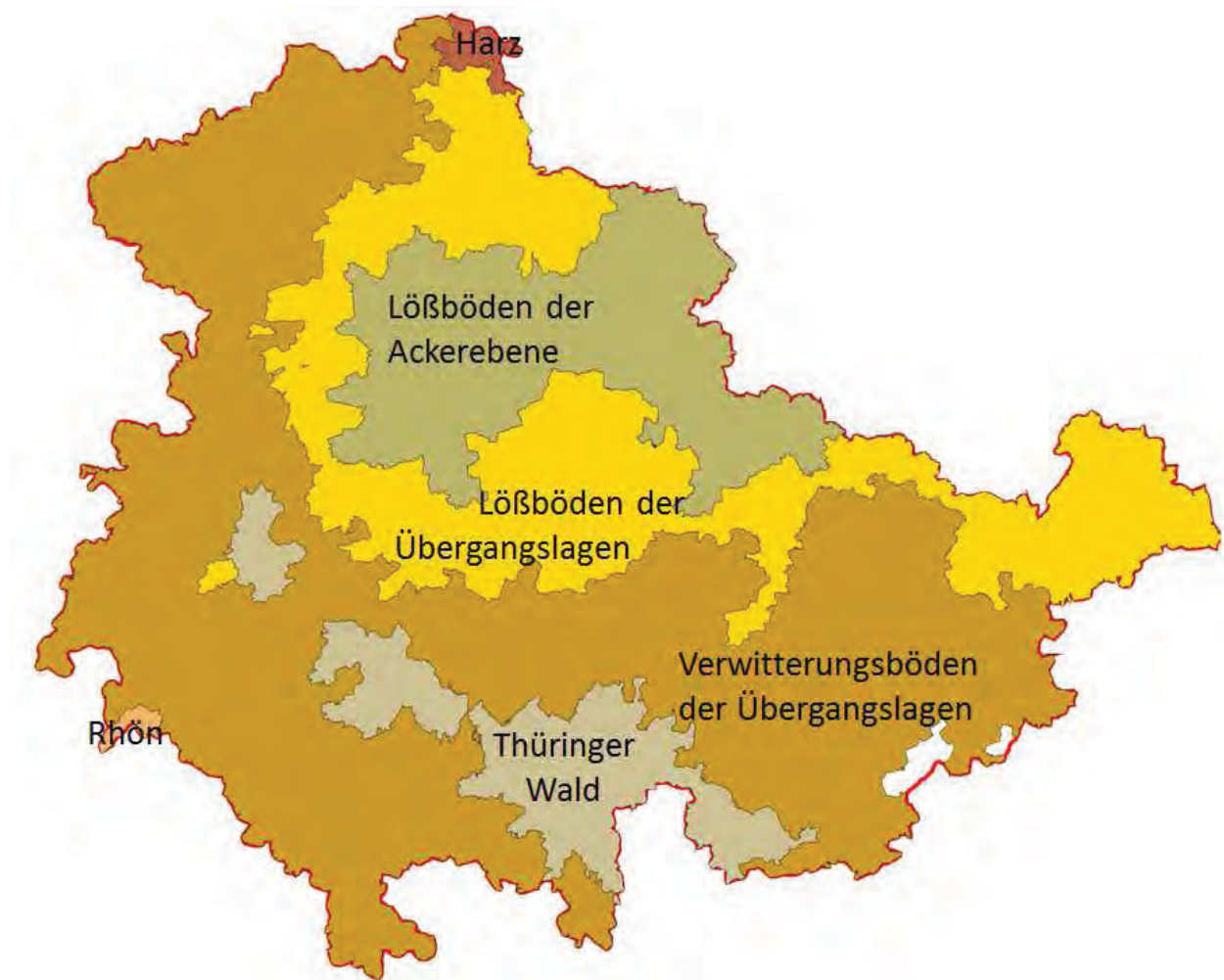
Abbildung 41: Boden-Klima-Räume/Anbaugebiete im Freistaat Thüringen
