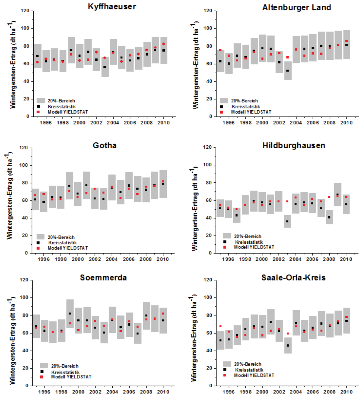
Abbildung 25: Vergleich statistischer Kreiserträge von sechs bodenklima- und anbaugiebts-repräsentativen Landkreisen des Freistaates Thüringen mit den mittels YIELDSTAT berechneten Kreiserträgen für Wintergerste im Zeitraum 1995-2010
