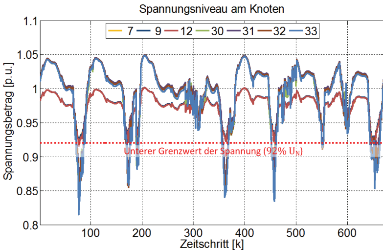
Bild 4.53: Verlauf Spannungsniveau bei Anwendung W2V im Szenario 2
