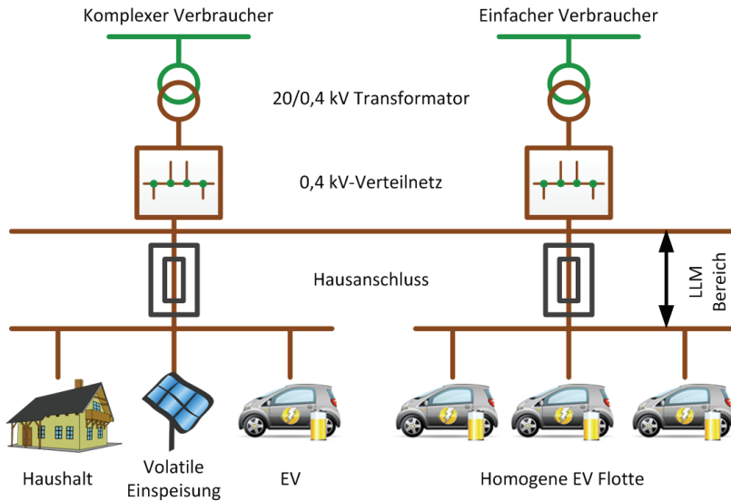
Bild 3.4: Komplexer und einfacher Verbraucher im Kontext Elektromobilität
