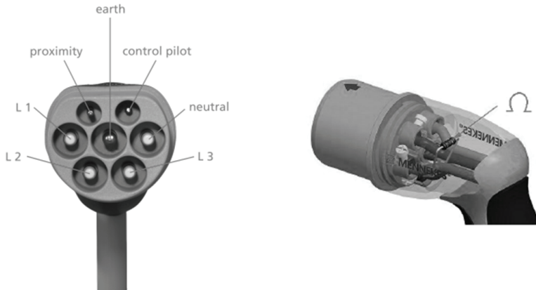
a) Design des Mennekes Steckers
