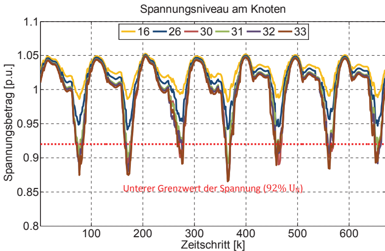
Bild 4.40: Verlauf Spannungsniveau bei Ungesteuerten Ladem im Szenario 1
