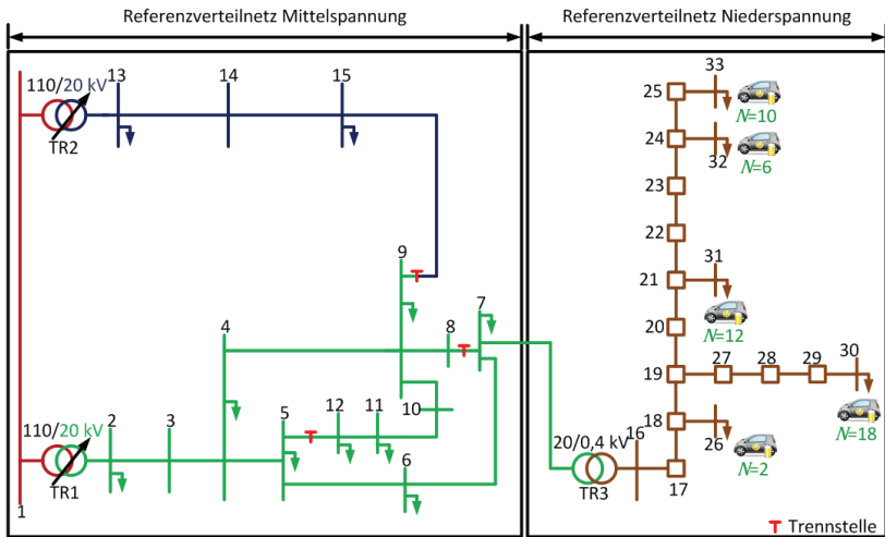
Bild 4.39: Verteilung EVs im Szenario 1
