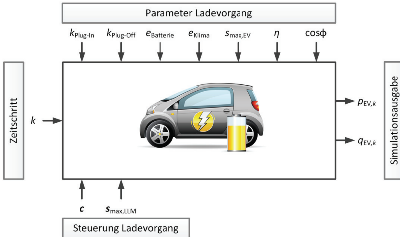
Bild 3.18: Übersicht allgemeines Modell eines EV zur Integration in eine Zeitreihensimulation zur Untersuchung der Beladung von EVs mittels stationärer Netzberechnung
