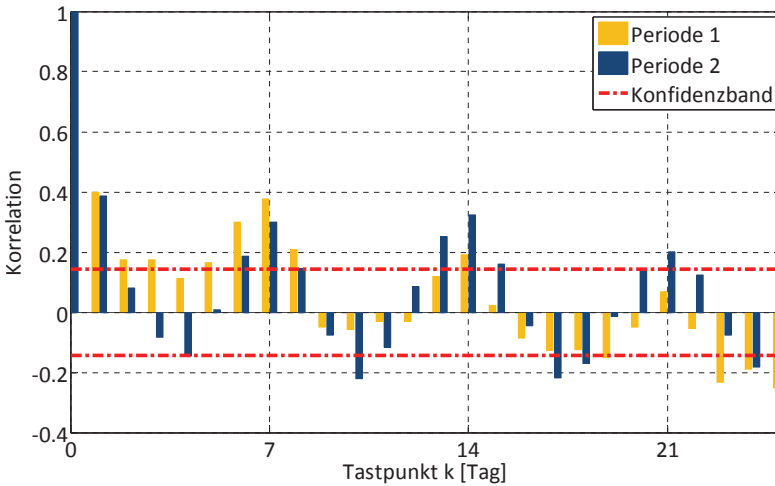
Bild 4.7: Autokorrelation der täglichen Energieaufnahme der Flotte
