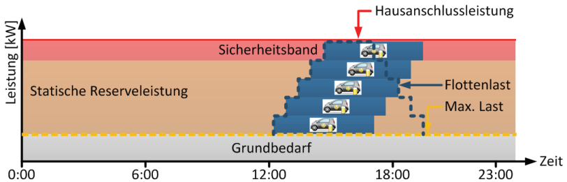
Bild 3.6: Nutzung der verfügbaren Leistung durch E-Fahrzeug Flotte
