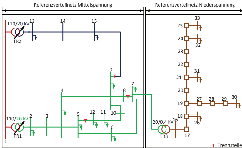
Bild 4.28: Übersicht des gewählten Referenzverteilernetzes für numerische Analysen
