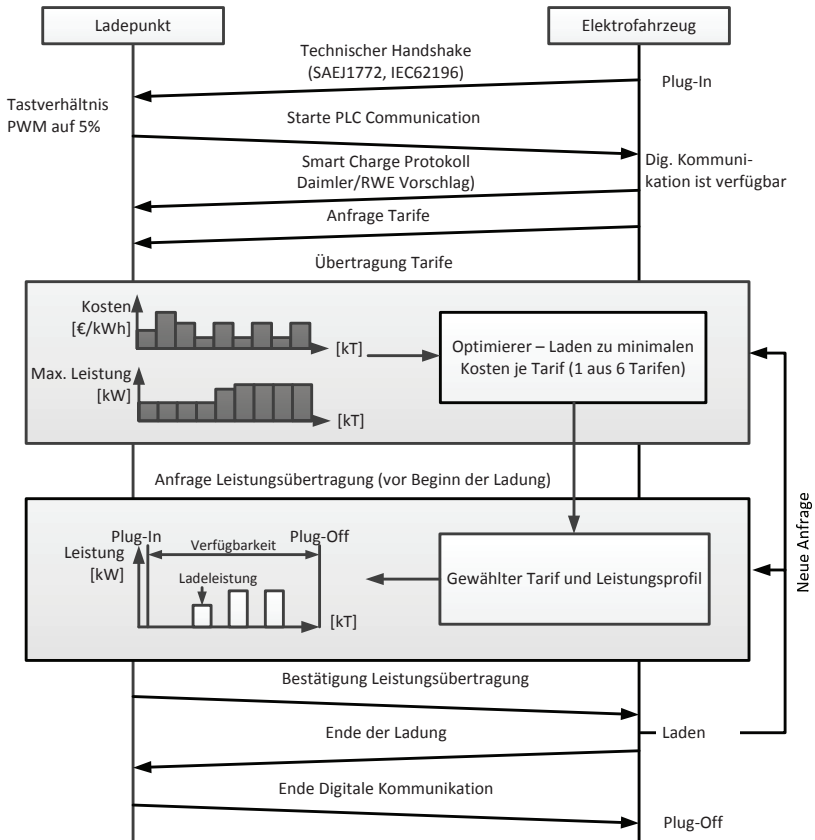
Bild 2.9: Informationsfluss zwischen Ladepunkt und EV nach [28], [65]
