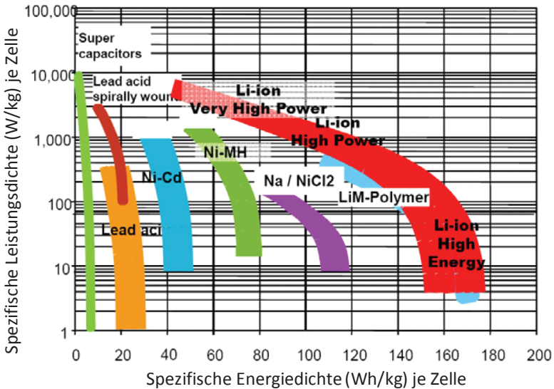
Bild 2.7: Ragone Diagramm von Batterietechnologien [59], [60], [61]
