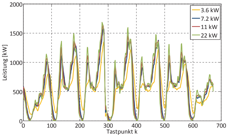
Bild 4.16: Lastprofile mit Klimatisierung (1935 Fahrzeuge, \cos\varphi=1 )
