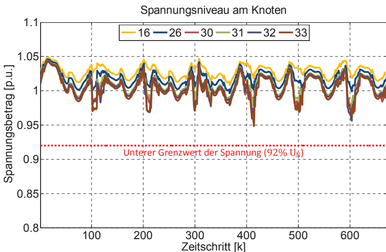
Bild 4.42: Verlauf Spannungsniveau bei Anwendung LLM ohne Ziel-funktion im Szenario 1
