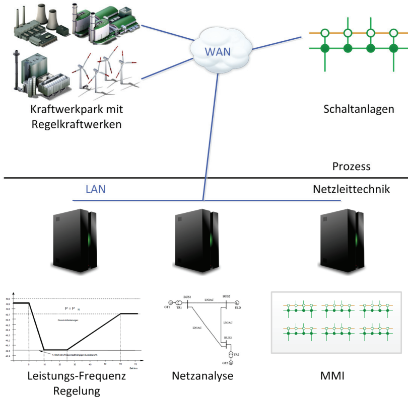
Bild 2.3: Prinzip Netzbetriebsführung von Übertragungsnetzen nach [19]
