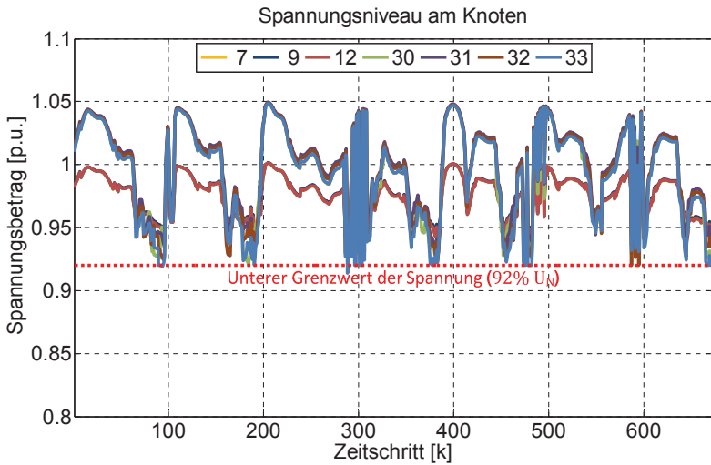
Bild 4.55: Verlauf Spannungsniveau bei Anwendung W2V und LLM im Szenario 2
