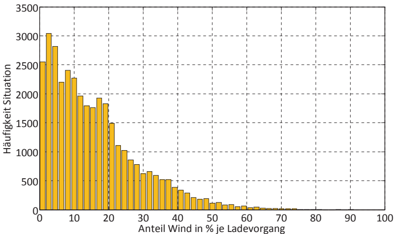
Bild 4.21: Häufigkeit Bereitstellungsquote Wind je 1/4 - Stunde 2009 in 50 Klassen (Daten sind entnommen von Referenz [88])
