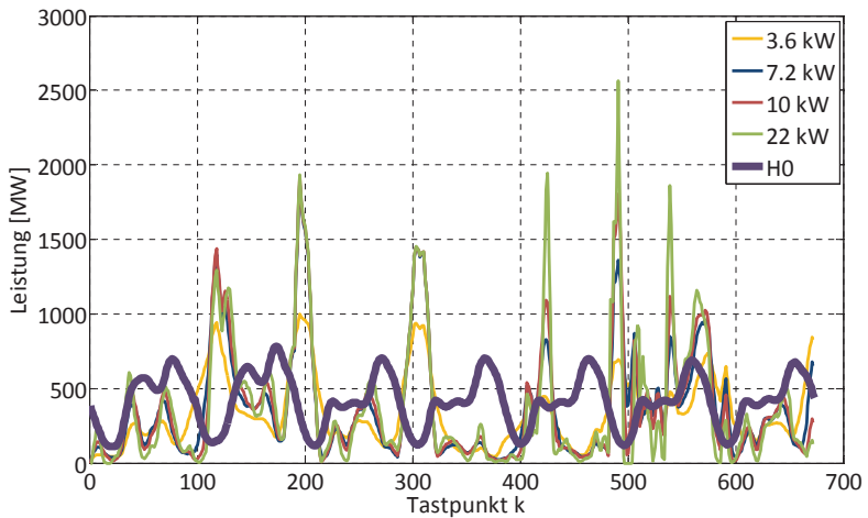
Bild 4.26: Lastprofil bei Nutzung gedrosselter Einspeisung (915.000 Fahrzeuge, \cos\varphi=1 )
