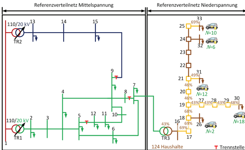
Bild 4.43: Belastung bei Anwendung LLM ohne Zielfunktion im Szenario 1
