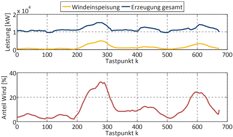
Bild 4.22: Einspeisesituation und Eingangssignal Steuerung Ladevorgänge (Daten sind entnommen von Referenz [88])
