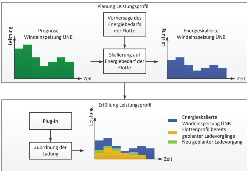
Bild 4.4: Grundprinzip windgesteuerten Ladens im Feldversuch
