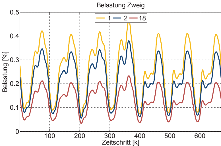
Bild 4.37: Belastung der Zweige ohne Elektrofahrzeuge
