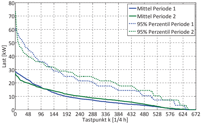
Bild 4.10: Geordnete Belastungskurve Wochenprofil
