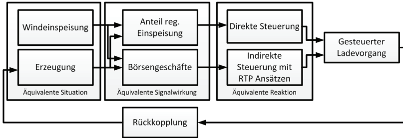
Bild 3.9: Ursache-Wirkungs-Prinzip Gesteuertes Laden W2V
