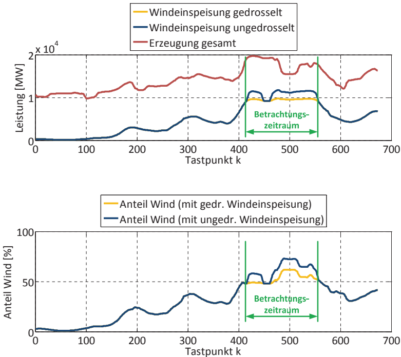
Bild 4.25: Gedrosselte und ungedrosselte Windeinspeisung
