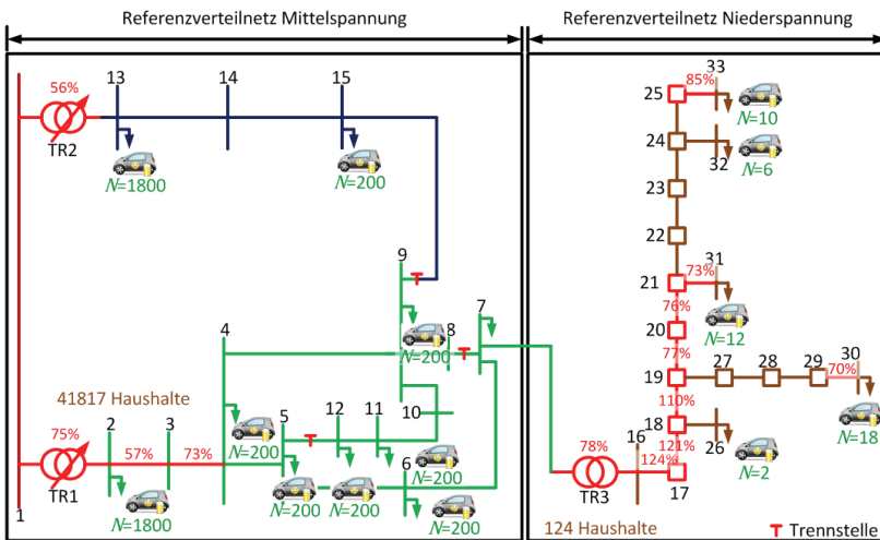
Bild 4.54: Überlastsituation bei Anwendung W2V im Szenario 2
