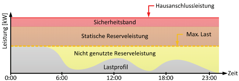
Bild 3.5: Ermittlung Reserveleistung für LLM für einen Haushalt
