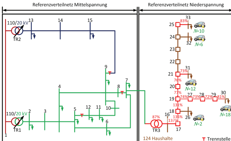
Bild 4.41: Überlastsituation bei Ungesteuerten Laden im Szenario 1
