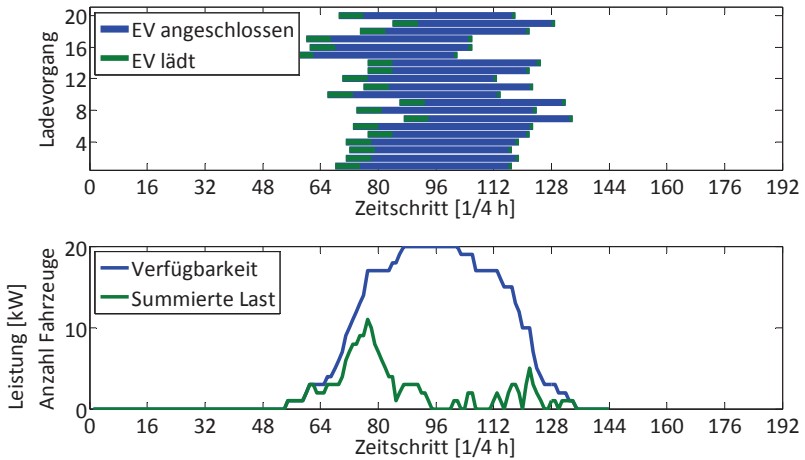
Bild 2.11: Beispielhafte Überlagerung von Ladevorgängen einer Flotte
