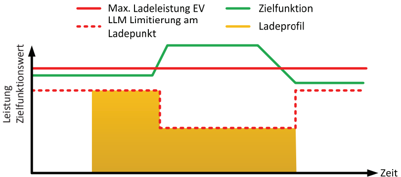
Bild 3.3: Beispiel optimierter Ladevorgang mit LLM Funktion
