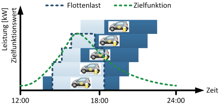
Bild 3.11: Beispielsituation synchronisierter Ladevorgänge
