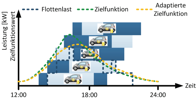
Bild 3.12: Beispielsituation Verwendung Neuberechnung Zielfunktion
