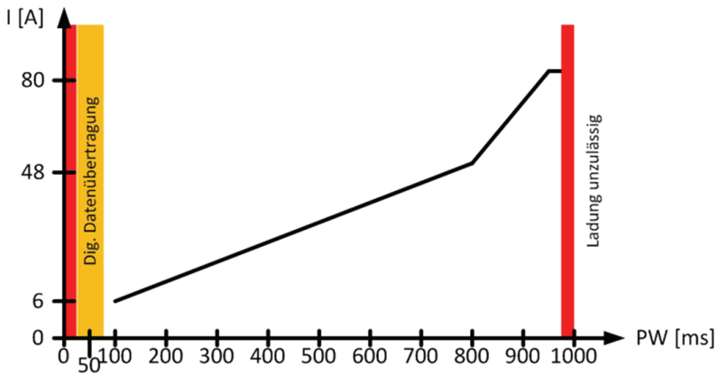
Bild 2.8: Pilotstromkreis und Kodierung des maximalen Ladestromes nach [46], [63]
