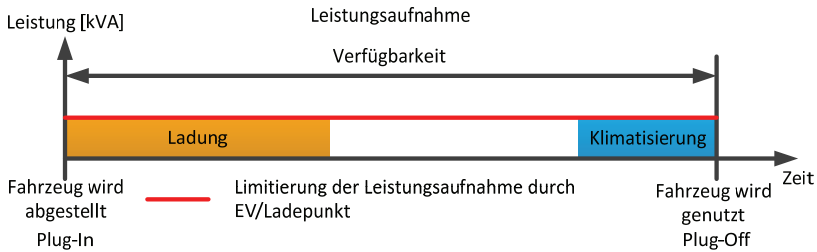
Bild 3.14: Ungesteuertes Laden mit Klimatisierung
