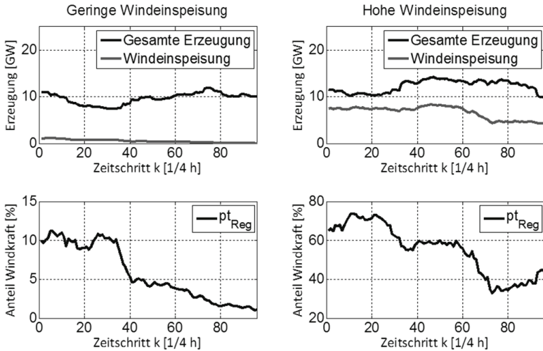
Bild 3.10: Verlauf pt_{\text{Reg}} für zwei Beispieltage (Daten sind entnommen von Referenz [88])
