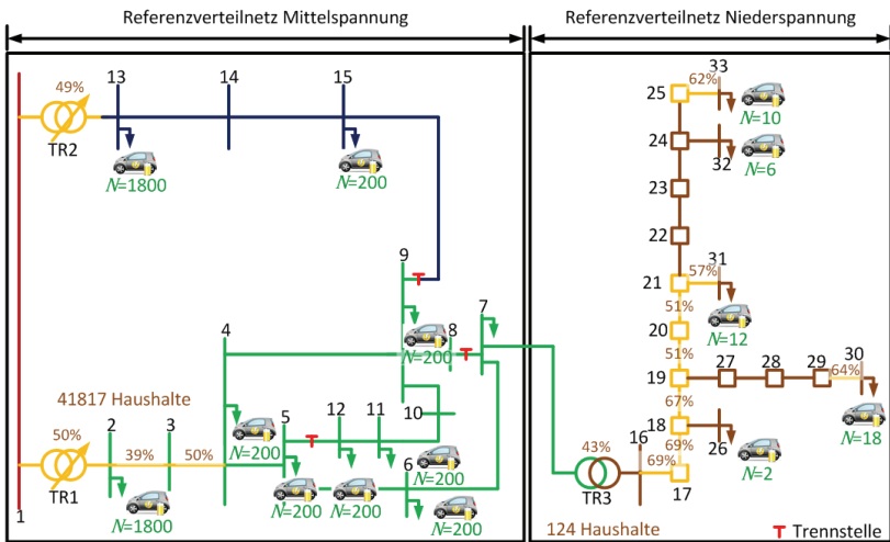
Bild 4.56: Maximalbelastung bei Anwendung W2V und LLM im Szenario 2
