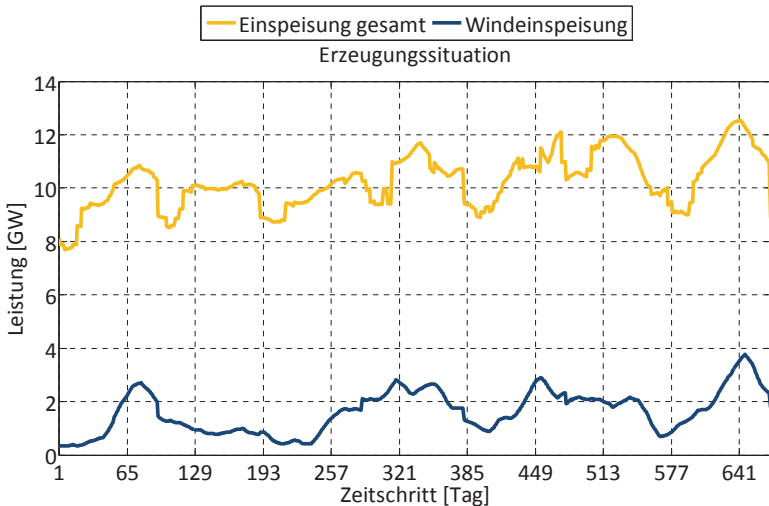
Bild 4.34: Einspeisesituation im Simulationshorizont (Daten aus Referenz [88] entnommen)
