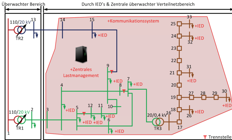
Bild 3.7: Verteilung IEDs im Verteilnetz
