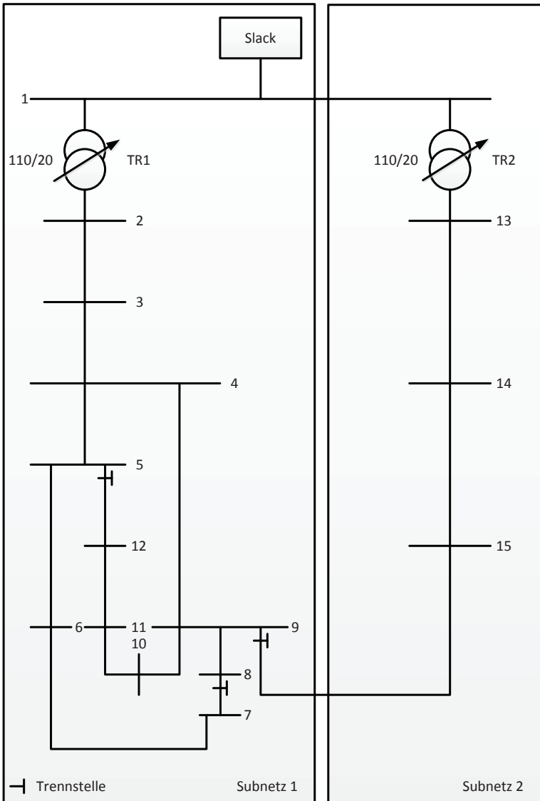
Bild A.3: MS Verteilerreferenznetz CIGRE TF C6.04.02 [85], [100]
