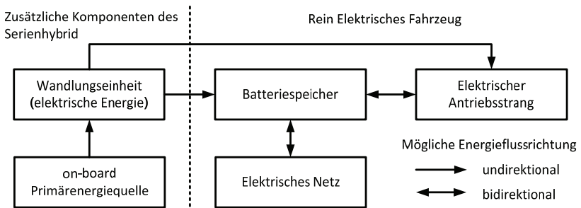
Bild 2.5: Energiefluss elektrischer Fahrzeuge [47], [48]
