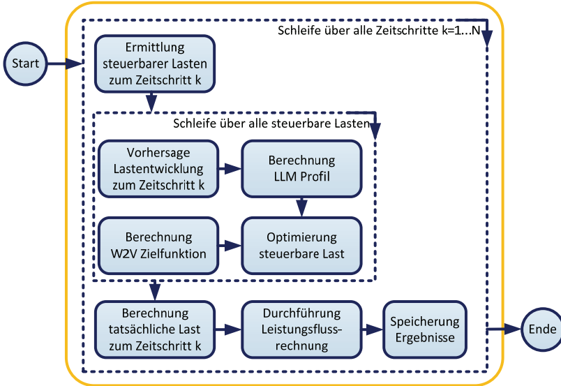
Bild A.5: Aktivitätsdiagramm Zeitreihensimulation
