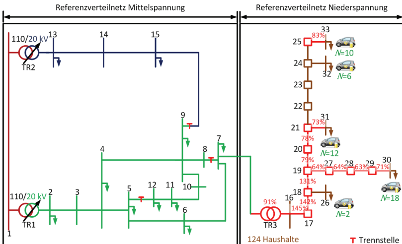
Bild 4.45: Überlastsituation bei Anwendung W2V im Szenario 1
