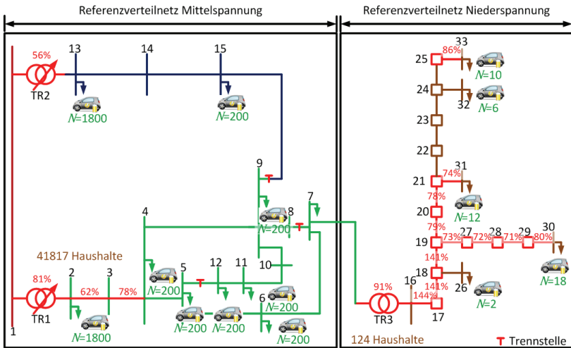
Bild 4.50: Überlastsituation bei Ungesteuerten Laden im Szenario 2
