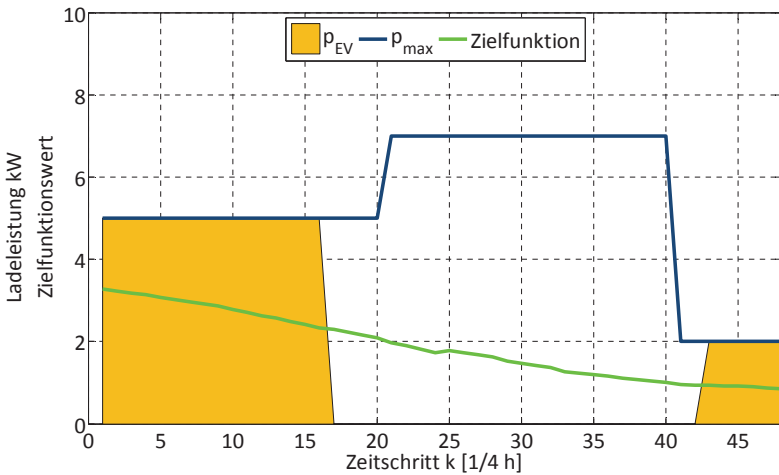
Bild 3.20: Beispiel gesteuerter Ladevorgang mit Klimatisierungsaufwand
