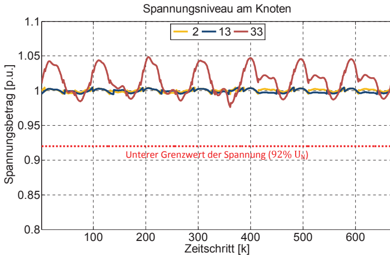
Bild 4.38: Spannungsniveau an den Knoten 2, 13, 33 ohne Elektrofahrzeuge
