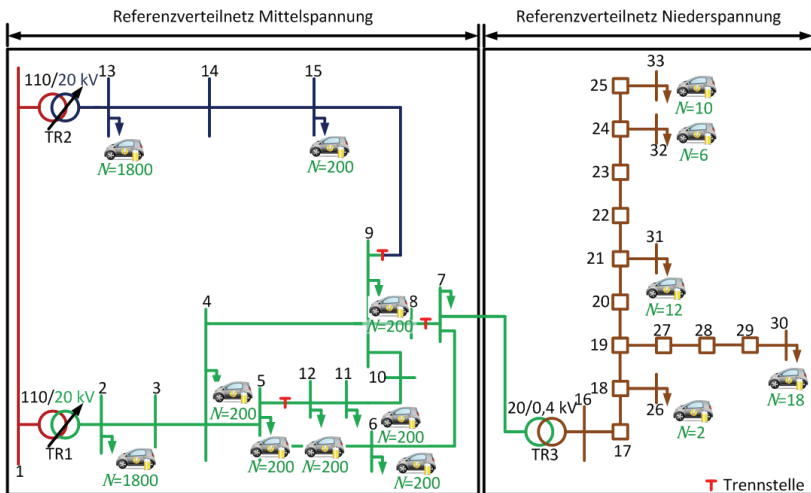
Bild 4.48: Verteilung EVs im Szenario 2
