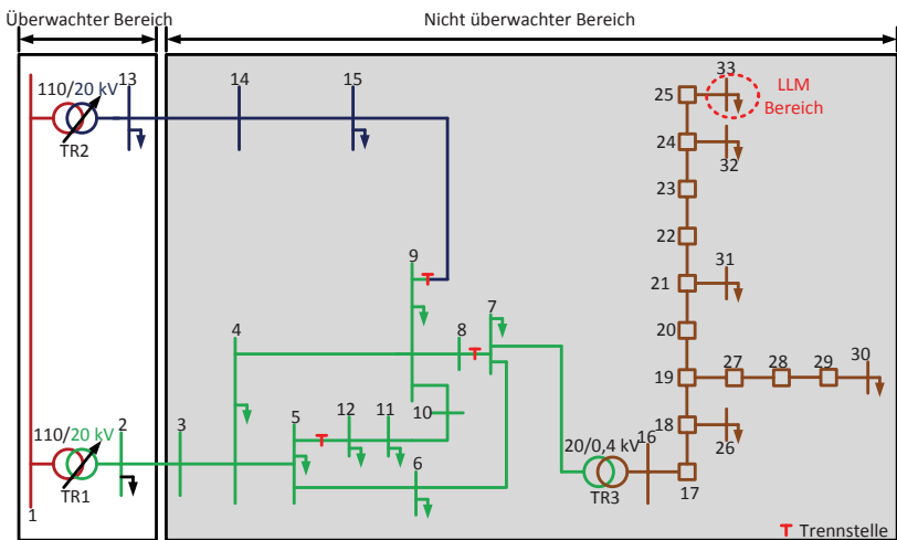
Bild 3.2: Lokalisation der LLM Funktionalität im definierten Referenzverteilnetz [85]
