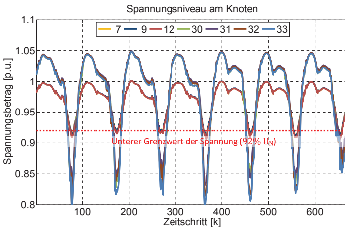
Bild 4.49: Verlauf Spannungsniveau bei Ungesteuerten Laden im Szenario 2
