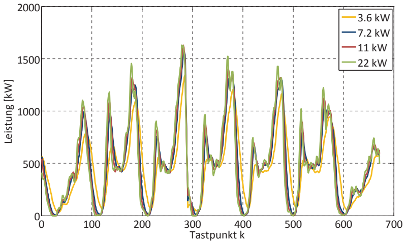
Bild 4.15: Lastprofile ohne Klimatisierung (1935 Fahrzeuge, \cos\varphi=1 )
