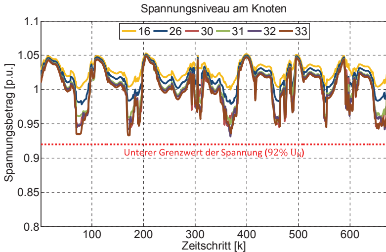
Bild 4.46: Verlauf Spannungsniveau bei synch. Ladung mit LLM im Szenario 1
