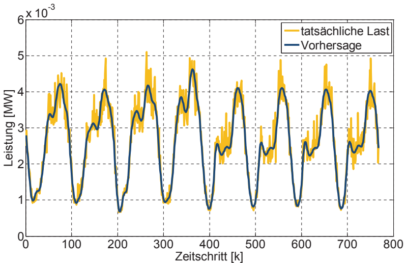
Bild 4.57: Vergleich Vorhersage und tatsächliche Last (einfache Unsicherheit)
