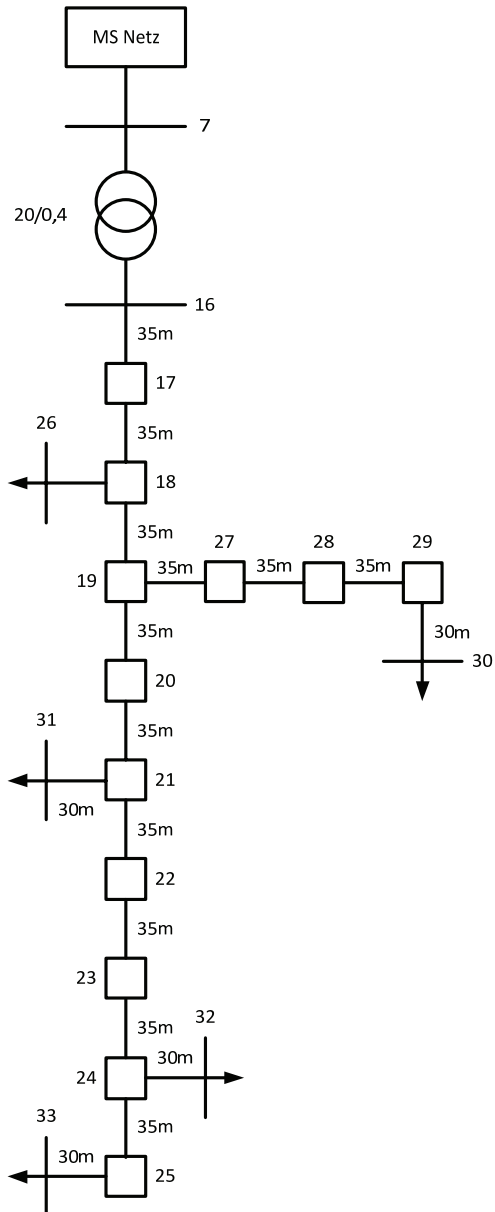
Bild A.4: NS Verteilerreferenznetz CIGRE TF C6.04.02 [85], [100]
