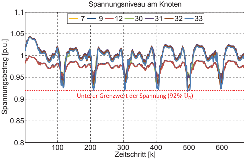
Bild 4.51: Verlauf Spannungsniveau bei Anwendung LLM ohne Ziel-funktion im Szenario 2
