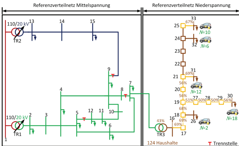
Bild 4.47: Belastung bei Anwendung W2V mit LLM
