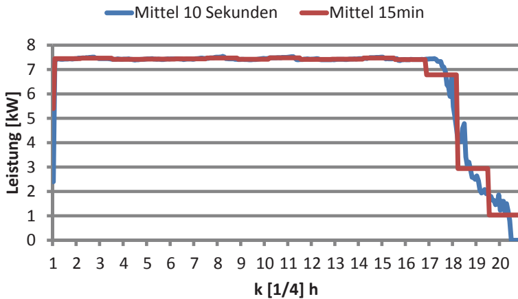
Bild 3.17: AC-seitige Messung einer Vollladung eines EV mit 7,2 kW Ladeleistung (Messung im Projekt Mini-E powered by Vat-tenfall)
