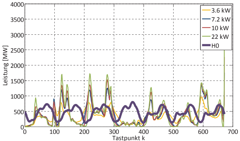
Bild 4.24: Konzentration Ladeleistung mit W2V große Flotte (915.000 Fahrzeuge, \cos\varphi=1 )
