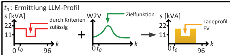
Bild 3.8: Bewertung zulässige Ladeleistung anhand Spannungsniveau und Betriebsmittelbelastung
