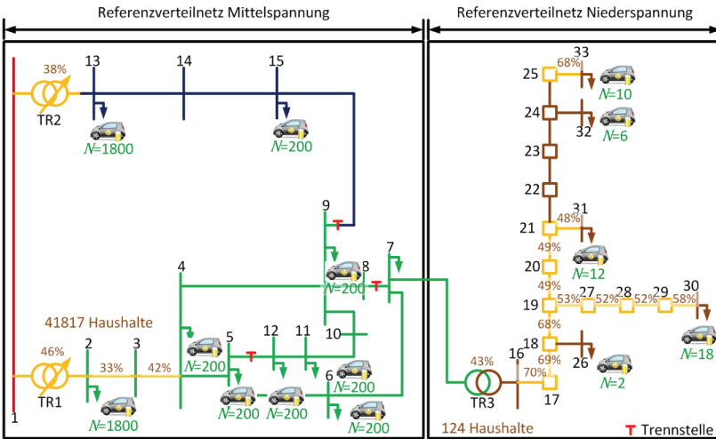
Bild 4.52: Belastung bei Anwendung LLM ohne Zielfunktion im Szenario 2
