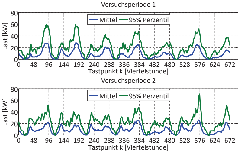
Bild 4.9: Wochenprofil Ungesteuerte Last Elektromobilität
