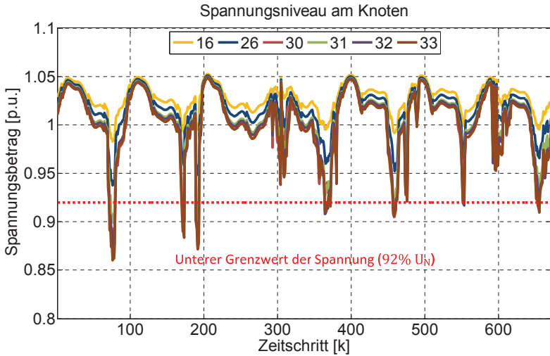
Bild 4.44: Verlauf Spannungsniveau bei Anwendung W2V im Szenario 1
