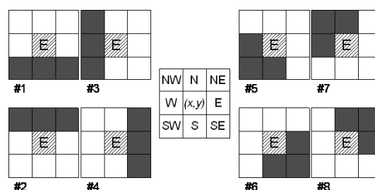
Fig. 1. Edge detection
